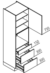
GBAK Geräteschrank für Backofen / Mikrowelle ↔ 60 ↑ 195/210/225 ↶ 60
