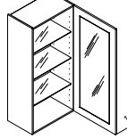
HAVDN Aufsatzschrank mit Glastür DN ↔ 45/50/60 ↑ 115/130/145 ↱ 35
