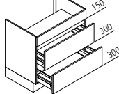
KAK-ML Kochstellenschrank für Muldenlüfter ↔ 60/80/90/100/120 ↑ 75 ↙ 60
