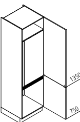
GK Geräteschrank für Kühlschrank / Nische 1780 mm ↔ 60 ↑ 195/210/225 ↱ 60
