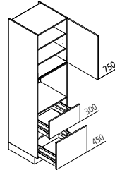
GBZ Geräteschrank für Backofen / Mikrowelle ↔ 60 ↑ 195/210/225 ↶ 60
