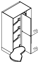
VELA Vorratsschrank- Ecke ↔ 110/115/125 ↑ 135/150 ↱ 60
