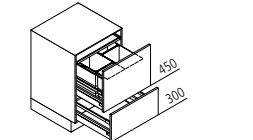
UABO Auszugsschrank mit Abfalleimer ↔ 30/40/45/50/60 ↑ 75 ↱ 60
