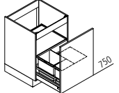
SABD Spülenunterschrank mit Abfalltrennsystem ↔ 45/50/60 ↑ 75 ↙ 60
