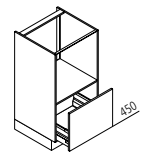
GBZ Geräteschrank für Backofen oder Mikrowelle ↔ 60 ↑ 105 ↱ 60
