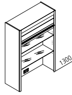
HAJGO Aufsatzschrank mit Jalousie in Glas-Optik ↔ 60/90 ↑ 115/130/145 ↱ 35/50/60 Lieferbar in Schwarz softmatt oder Schwarz Hochglanz
