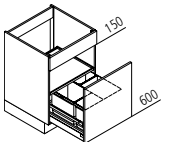
SAB Spülenunterschrank mit Abfalltrennsystem ↔ 45/50/60/80/90/100/120 ↑ 75 ↙ 60
