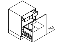
UABDG Auszugsschrank mit Abfalleimer ↔ 40/45/50/60 ↑ 75 ↱ 60
